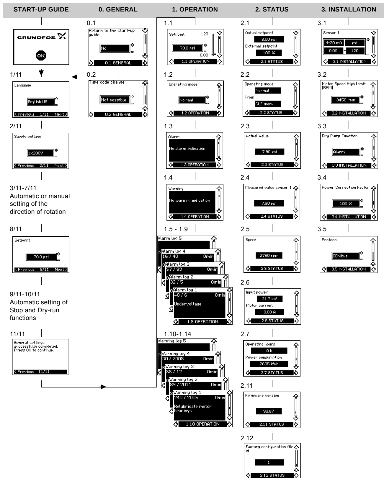
Fig. 23 Menu overview
