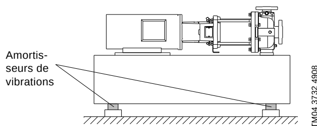
Fig. 9 Pompe sur amortisseur de vibrations
